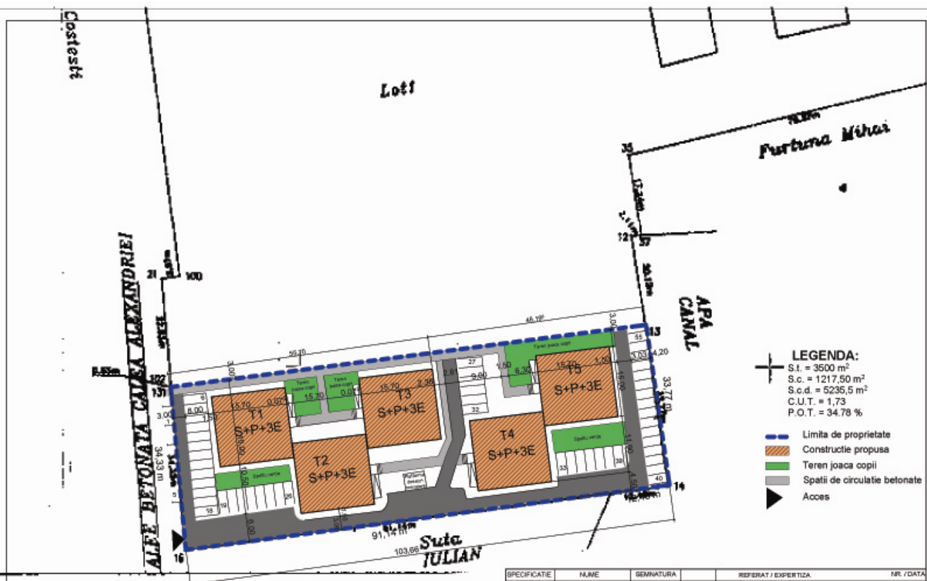
PLAN DE SITUATIE sc. 1:500
